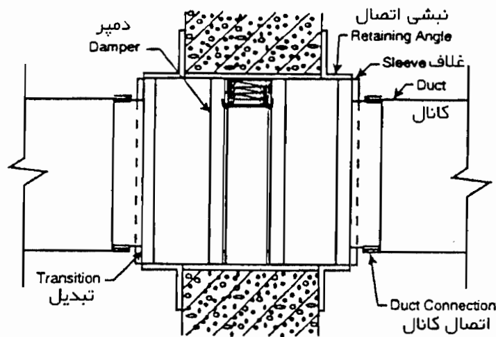
۹-۵-۴-۲ پلنوم (PLENUM)
