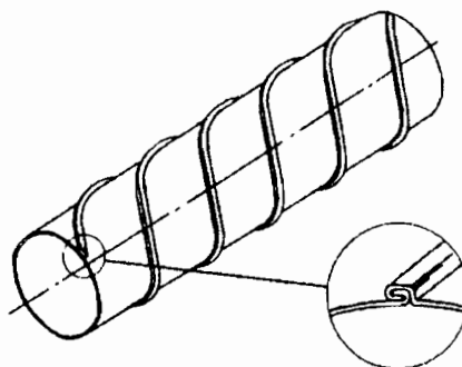
شکل شماره (۳-۶-۴-۲) "ب" (۱) ساخت و اتصال درز در کانال‌های گرد مارپیچ
