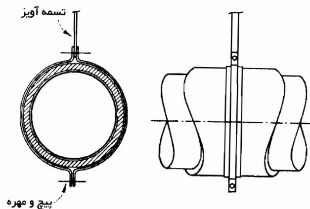
شکل شماره (۴-۸-۴-۲) "ب" (۲) آویز و بست کانال گرد افقی، بست خارج از عایق
