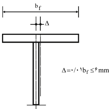
شکل ۱۰-۴-۳ رواداری محل اتصال جان به بال.
