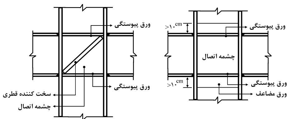
شکل ۱۰ - ۲ - ۲۳ نمایش سخت کننده های قطری و ورق مضاعف در چشمه اتصال.
