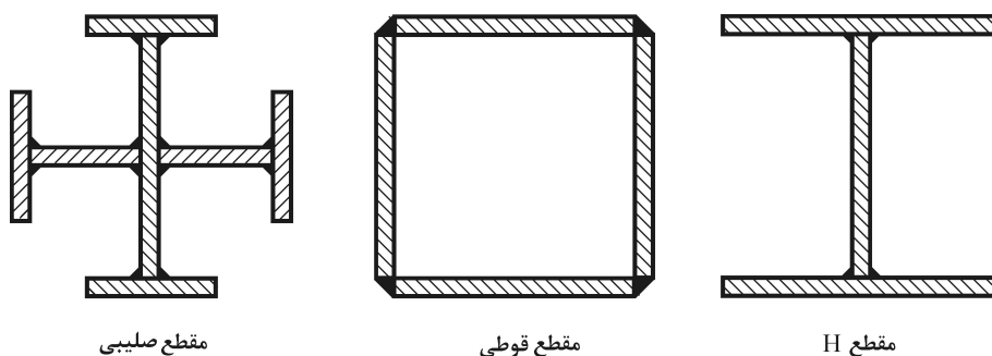
شکل ۱۰-۲-۴-۷ مقاطع اعضای فشاری ساخته شده از ورق.
