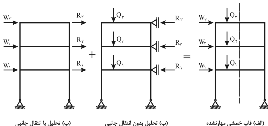
شکل ۱۰-۲-۷-۴ تحلیل قاب بدون و با انتقال جانبی.
