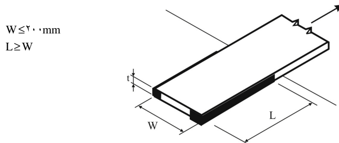
شکل ۱۰-۲-۴ جوش گوشه در انتهای تسمه‌های کششی.
