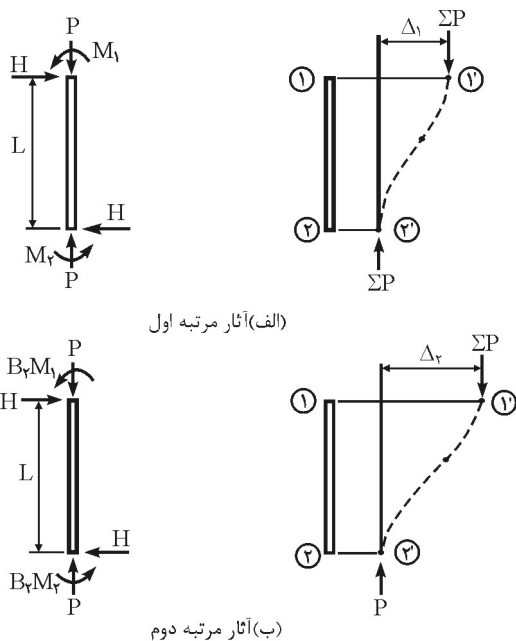
شکل ۱۰-۷-۲-۱ آثار مرتبه اول و آثار مرتبه دوم.
