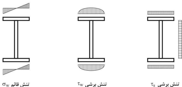
شکل ۱۰-۱-۸-۱ توزیع تنش در مقاطع I شکل تحت اثر لنگر پیچشی.
