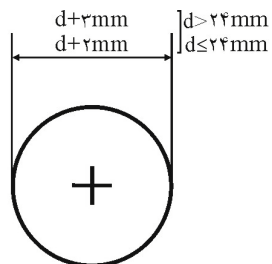
سوراخ استاندارد (اتصالات اتکایی و اصطکاکی)
