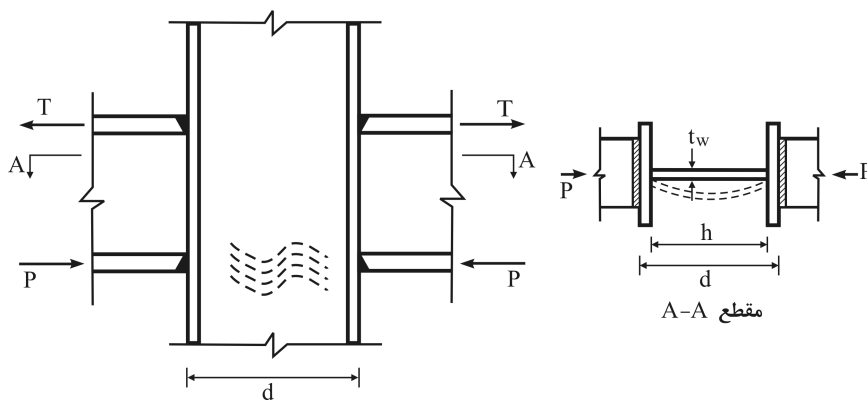
شکل ۱۰-۲-۱۰-۲۱ کمانش فشاری جان در مقابل یک جفت نیروی متمرکز فشاری.
