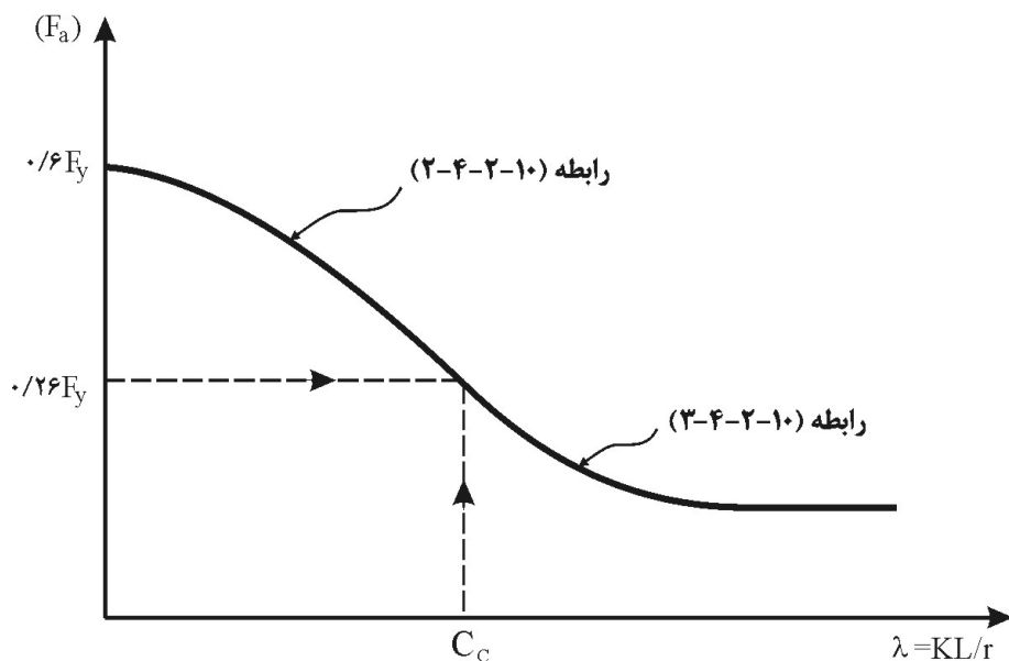
شکل ۱۰-۴-۱ نمودار تغییرات تنش فشاری مجاز برحسب لاغری حداکثر.
