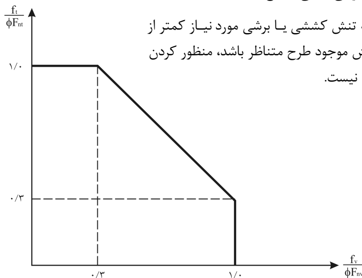
شکل ۹ - ۱۰ - ۲ - ۱۰ اثر متقابل کشش و برش در اتصالات اتکایی.
