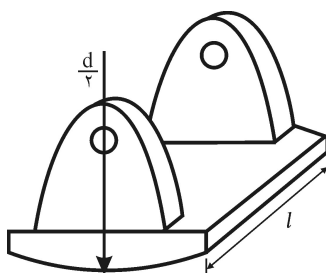
شکل ۱۰-۲-۱۵ کفشک‌های تکیه‌گاهی.
