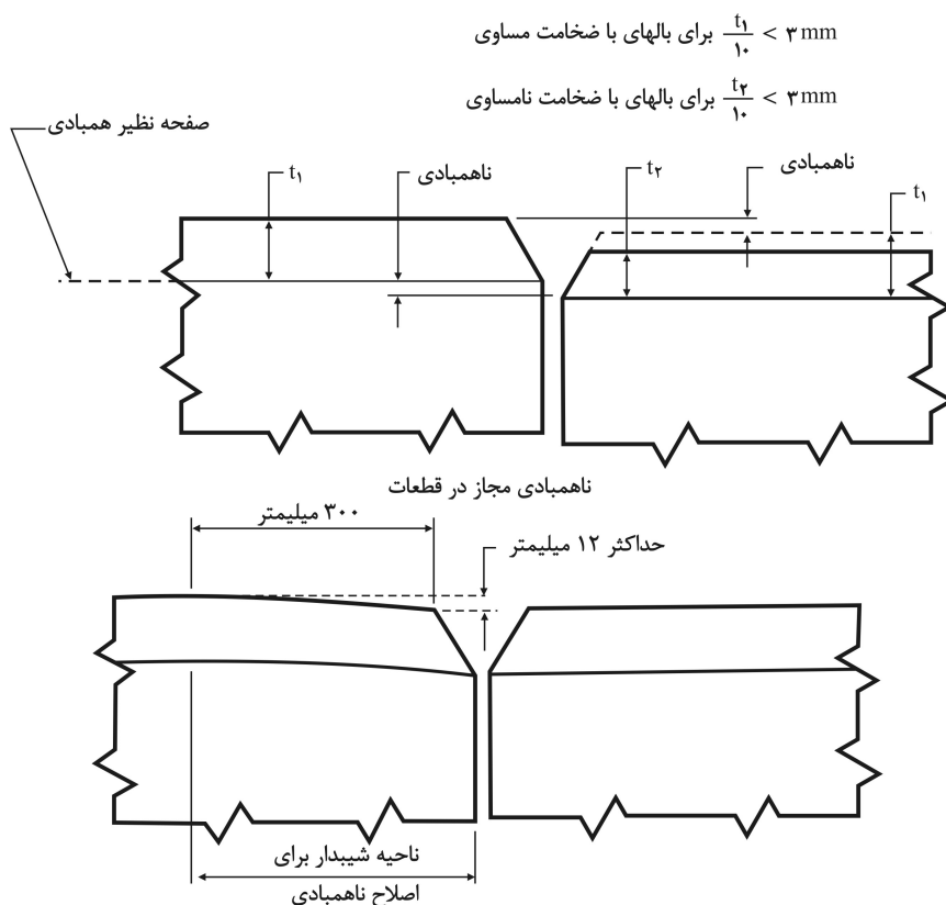
شکل ۱۰ - ۴ - ۲ اصلاح ناهمبادی و ناهم محوری.
