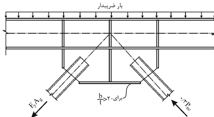
شکل ۱۰-۳-۹ ب نیروی غیرمتعادل مهارنده‌های کششی و فشاری، در طراحی به‌روش حالات حدی.
