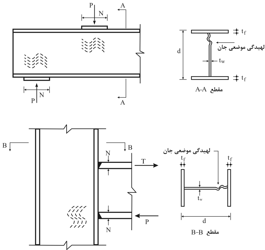
شکل ۱۰ - ۲ - ۱۰ - ۱۹ لهدگی جان در مقابل نیروی متمرکز فشاری.
