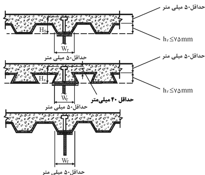
شکل ۱۰-۹-۱ محدودیت‌های ورق دوزنقه‌ای در تیرهای مختلط.
