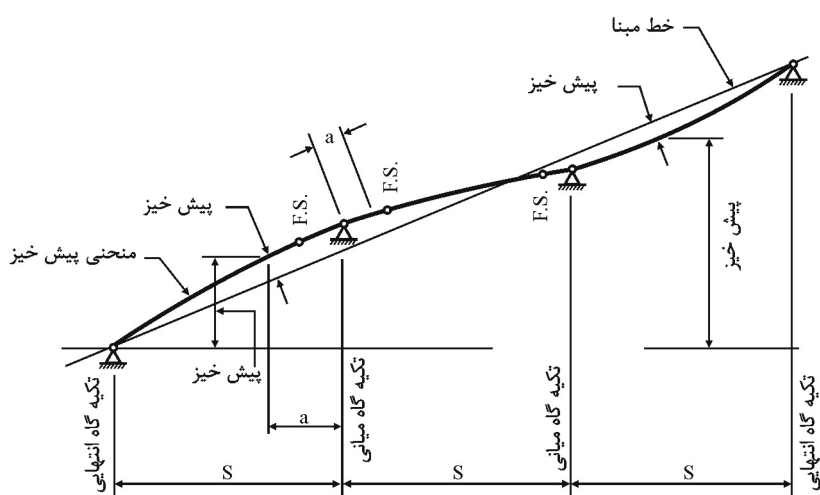
نمای جانبی پیش نصب تیر
