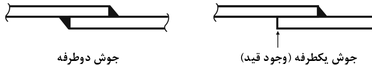
شکل ۱۰-۲-۳ وجود قید در جوش گوشه اتصالات پوششی (رویهم).
