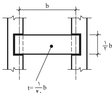
شکل ۱۰-۲-۳-۳ هندسه قیدهای موازی.
