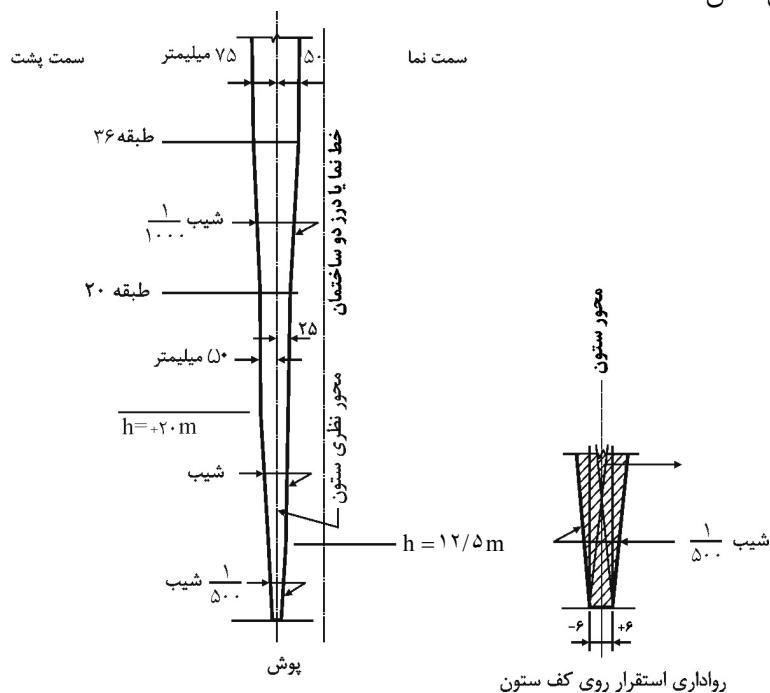
شکل ۹-۴-۱۰ پوش بدشاقولی ستون.
