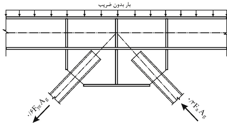
شکل ۱۰-۳-۹ الف نیروی غیرمتعادل مهارنده‌های کششی و فشاری در طراحی به‌روش تنش مجاز.
