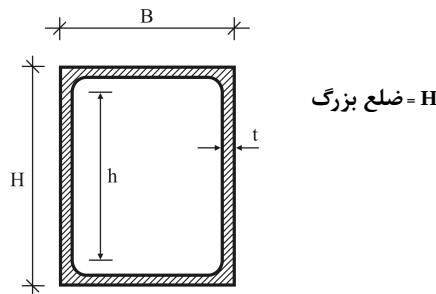
شکل ۱۰-۲-۸-۱ مقطع قوطی شکل.
