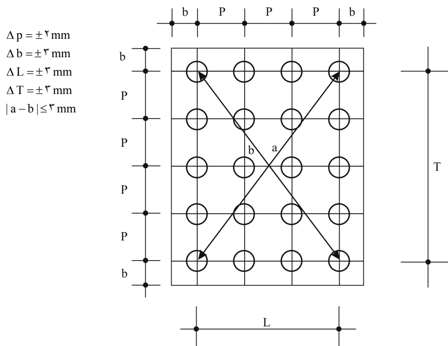
شکل ۱۰-۴-۱۲ رواداری سوراخ‌های پیچ.
