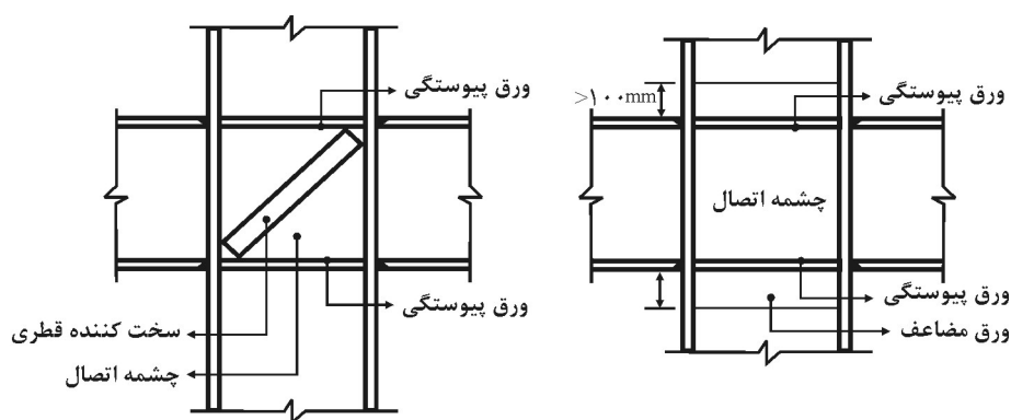
شکل ۱۰-۱-۱۱-۳ نمایش سخت کننده‌های قطری و ورق مضاعف در چشمه اتصال.
