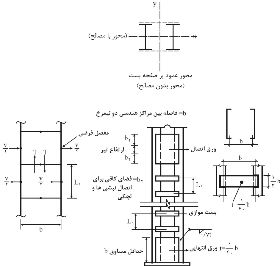
شکل ۱۰-۱-۴-۵ ستون با بست های موازی
