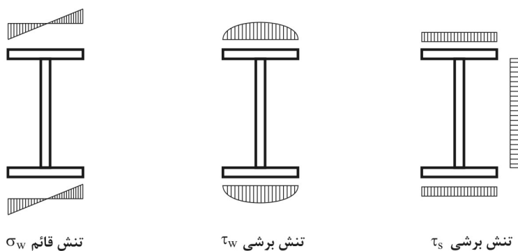
شکل ۸-۲-۱۰ توزیع تنش در مقاطع I شکل تحت اثر لنگر پیچشی.
