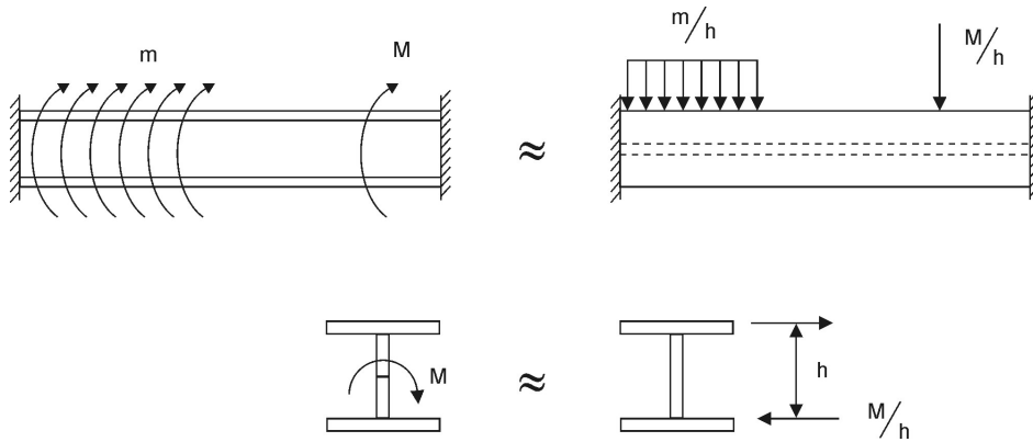
شکل ۱۰-۱-۸-۲ روش تشبیه پیچش به خمش.
