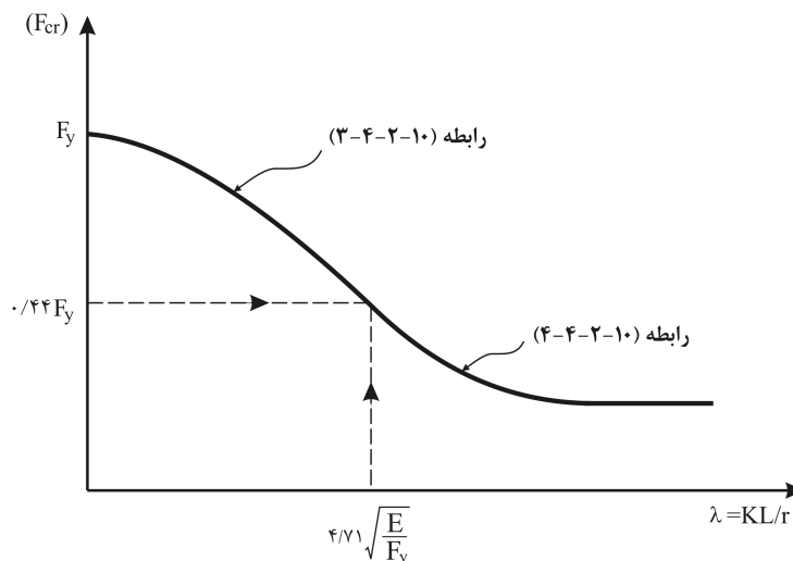
شکل ۱۰-۲-۴-۱ رابطه F_{cr} با نسبت لاغری \lambda برای اعضای فشاری براساس کمانش خمشی.
