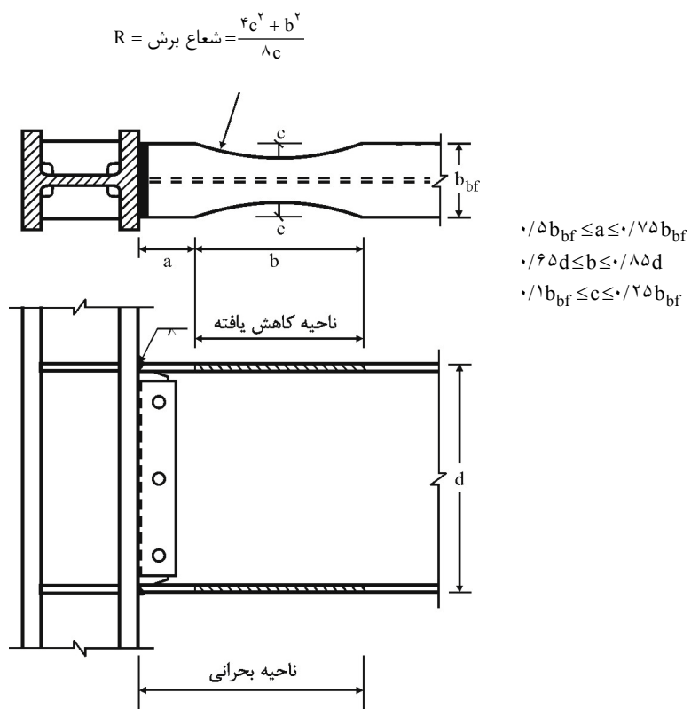
شکل ۱۰- ۳- ۷ (ت) اتصال صلب مستقیم تیر با مقطع کاهش یافته در قاب‌های شکل پذیری متوسط و زیاد.
