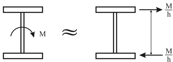
شکل ۱۰-۲-۸-۳ روش تشبیه پیچش به خمش.
