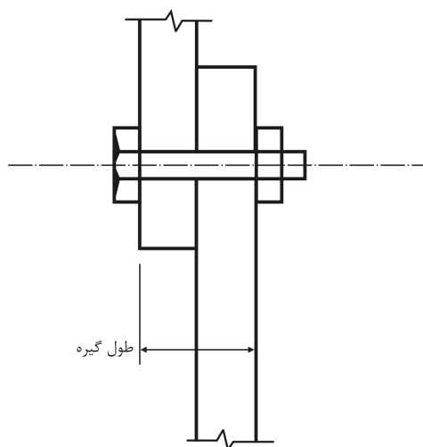
شکل ۱۰-۲-۸ طول گیره وسایل اتصال.
