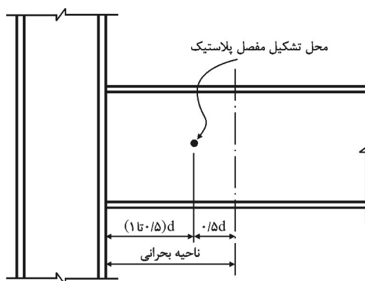
شکل ۱۰-۳-۴ ناحیه بحرانی در دو انتهای تیر.
