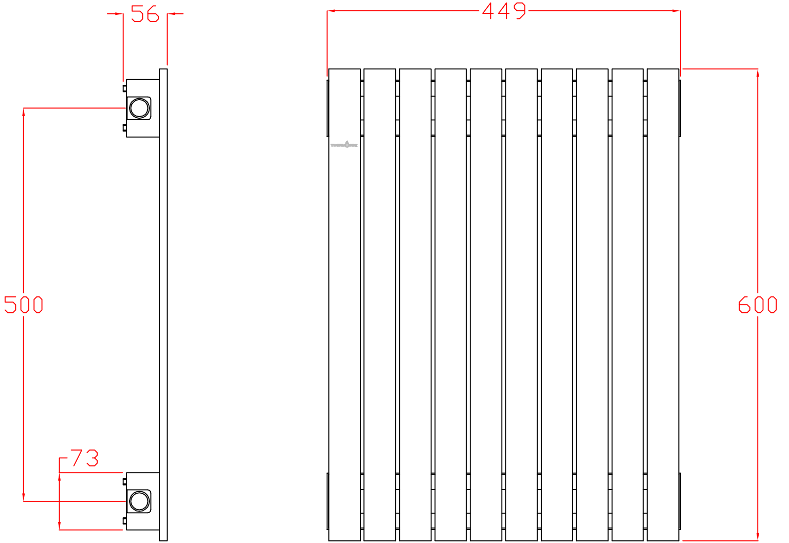
Thermobox ® TX10 dimensions
