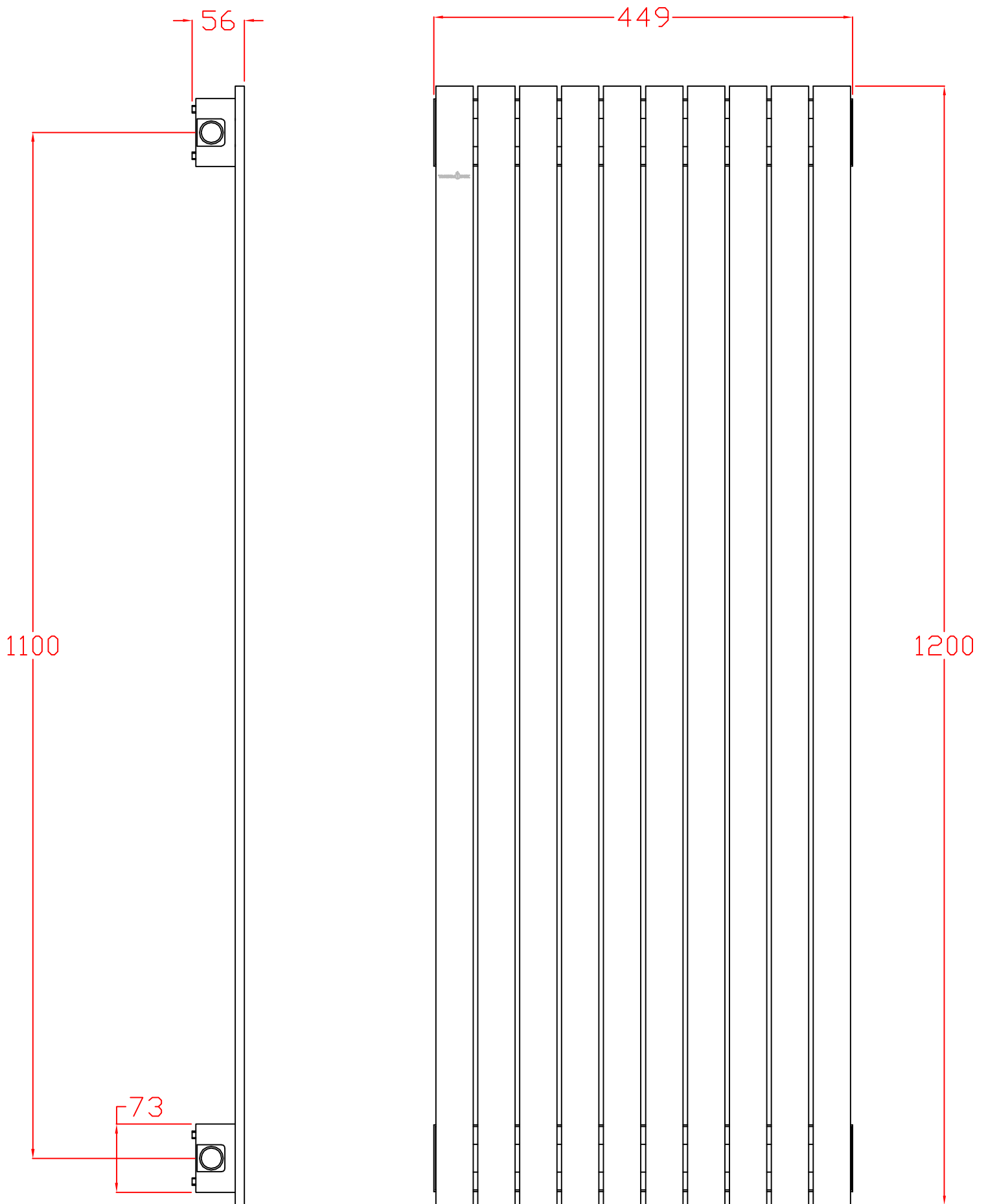
Thermobox ® TX10L dimensions
