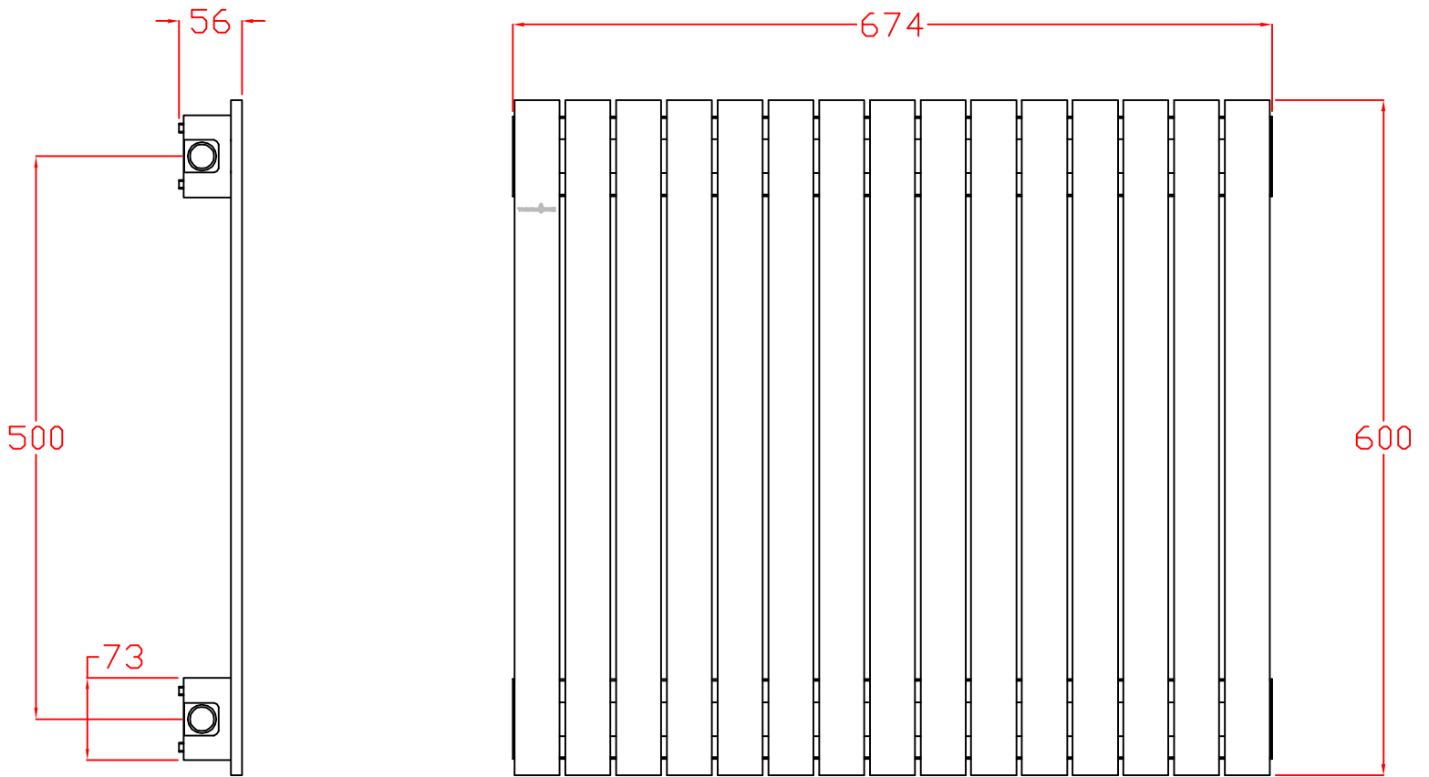
Thermobox ® TX15 dimensions
