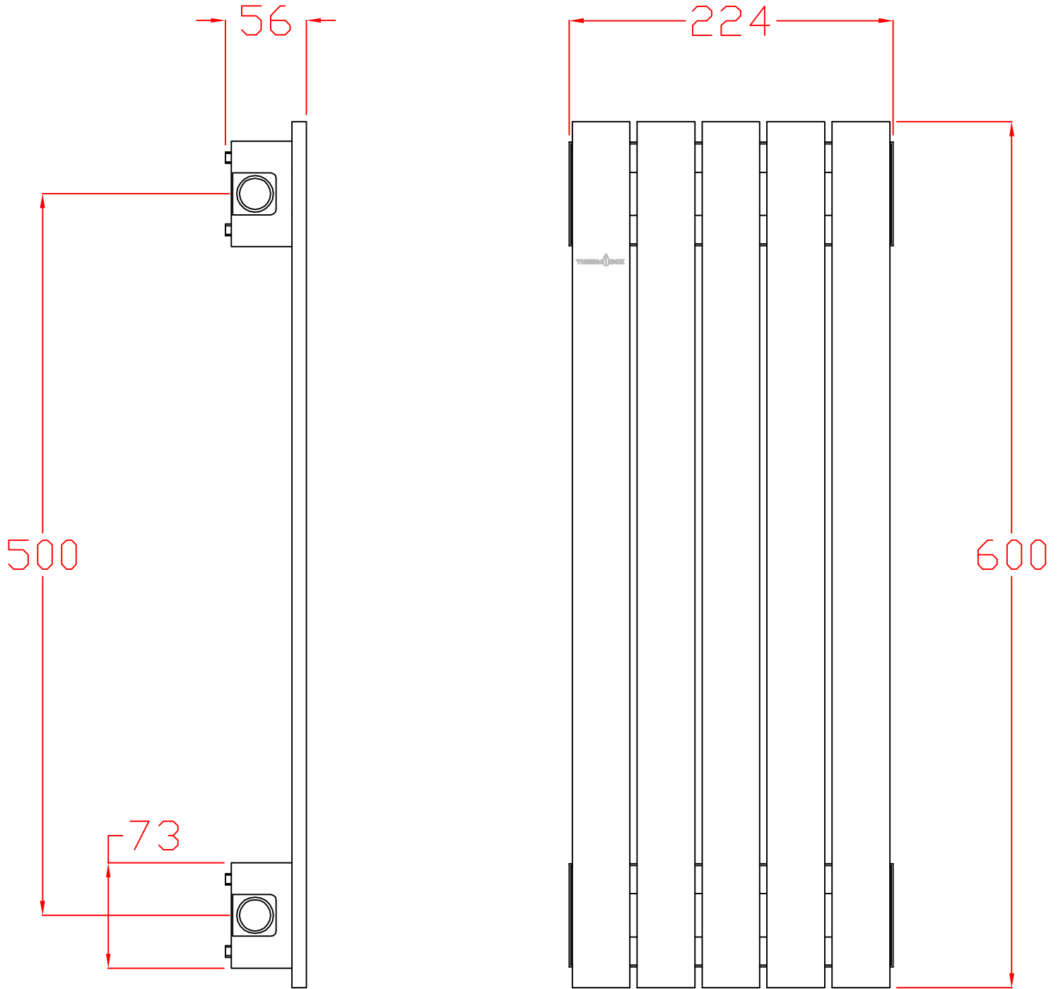
Thermobox ® TX5 dimensions
