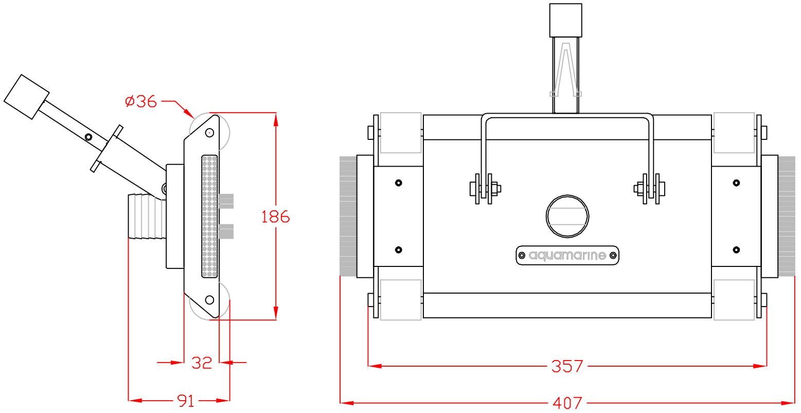
Aquamarine ® sweeper haed dimensions
